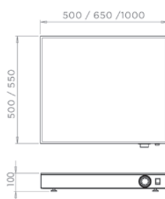
MEDIDAS PLACA CALIENTE SOBREMESA
