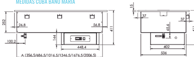
MEDIDAS CUBA BAÑO MARÍA
