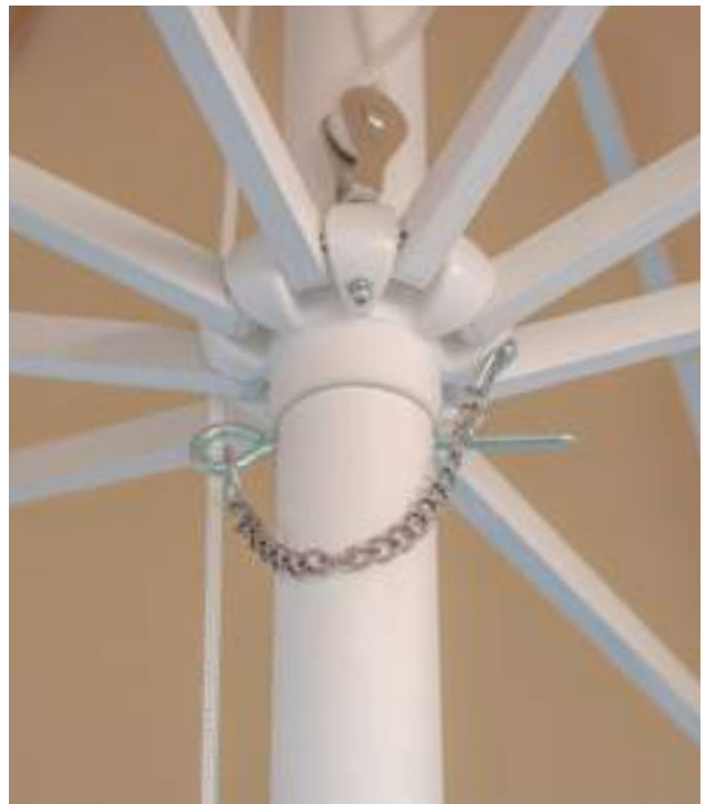
Sistema de apertura por polea y bloqueo de seguridad con pasador / Pulley system with safety pin lock / Système de poulie, avec goupille de sécurité
